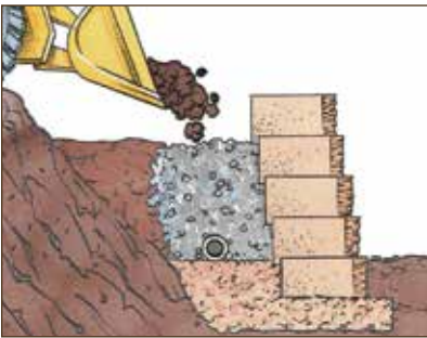
Diagram 5—Backfill
