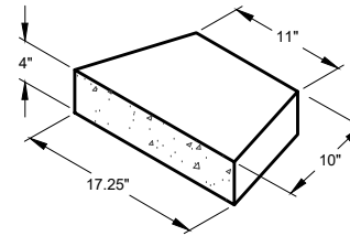
CAP UNIT
